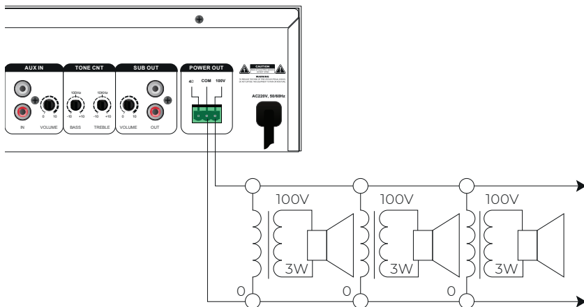
Рисунок 3 – Подключение громкоговорителей в режиме 100 В
