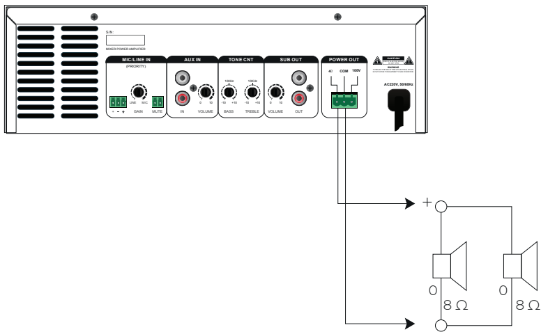
Рисунок 4 – Подключение громкоговорителей в режиме 4 Ом
